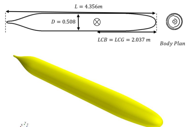
شکل ۱- هندسه شناور مدل سابوف بدون متعلقات
