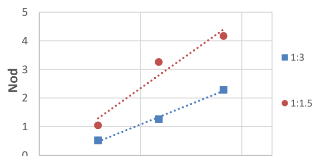
شکل ۱۱ - تأثیر شیب پیشانی بر پایداری پنجه
