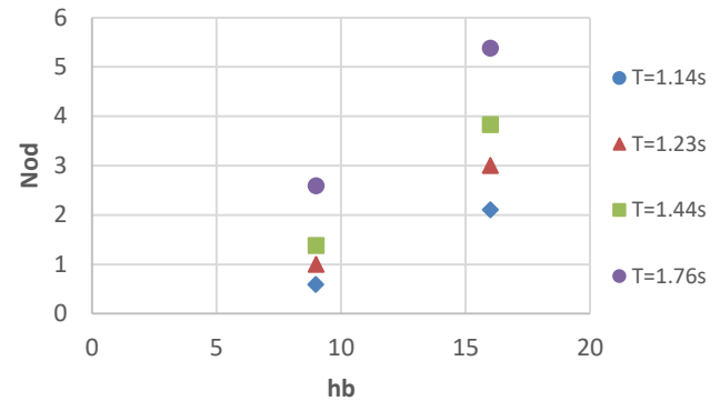
شکل ۷ - تاثیر پارامتر تراز سکو از سطح ایستابی بر پایداری پنجه
