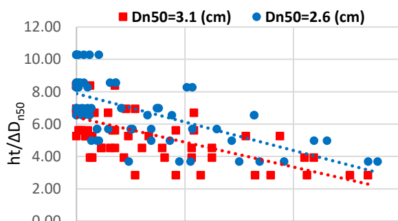
شکل ۹ - تاثیر قطر اسمی بر افزایش آسیب
