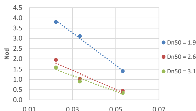
شکل ۱۰ - نمودار آسیب وارد شده به پنجه براساس تیزی موج برای سه قطر اسمی متفاوت
