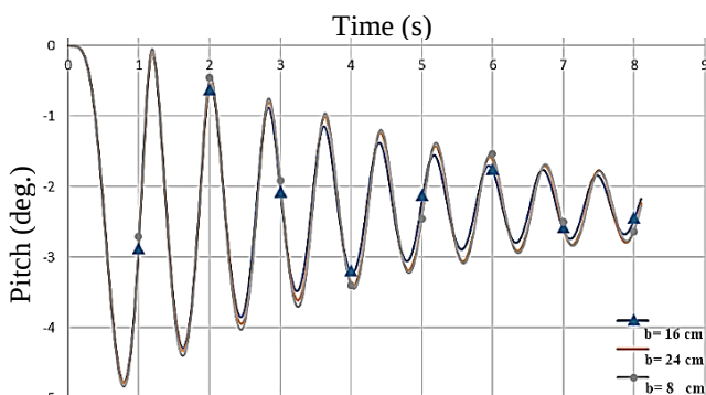
شکل ۱۶- نمودار حرکت پیچ شناور با پایدارساز هیدروفوبیلی زاویه‌دار با سه عرض میانی مختلف
