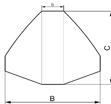
شکل ۸- نمای از بالای هیدروفویل زاویه‌دار
