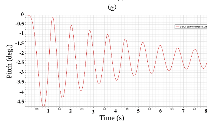
شکل ۱۴- نمودار حرکت پیچ شناور با پایدارساز هیدروفوبیلی زاویه‌دار با سه عرض میانی مختلف؛ (الف): کم ( b = 8 \text{ cm} ), (ب): متوسط ( b = 16 \text{ cm} ), (ج): زیاد ( b = 24 \text{ cm} )
