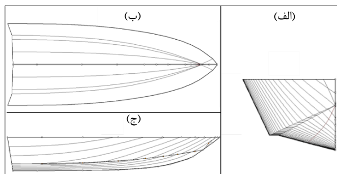
شکل ۷- خطوط بدنه شناور سُرسی تک بدنه نمونه با نمای مختلف؛ (الف): نمای نیم‌بدنه از جلو، (ب): نمای بالا، (ج): نمای راست.
