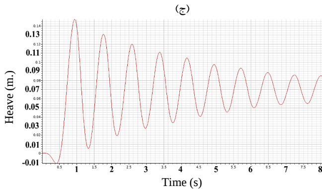
شکل ۱۵- نمودار حرکت هیو شناور با پایدارساز هیدروفوبیلی زاویه‌دار با سه عرض میانی مختلف؛ (الف): کم ( b = 8 \text{ cm} ), (ب): متوسط ( b = 16 \text{ cm} ), (ج): زیاد ( b = 24 \text{ cm} )
