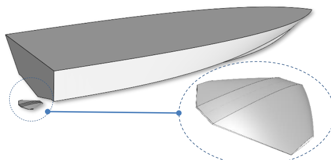
شکل ۹- مدل سه‌بعدی شناور با پایدارساز هیدروفویلی زاویه‌دار و نمایش سه‌بعدی بزرگنمایی پایدارساز زاویه‌دار
