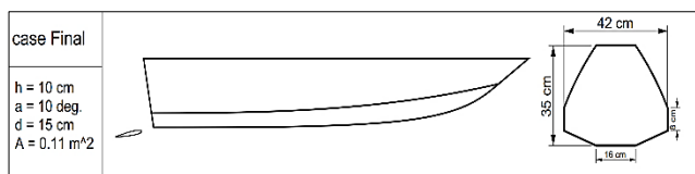
شکل ۲۱ - پارامترهای پایدارساز هیدروفویلی نهایی شناور
