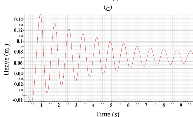
شکل ۱۹- نمودار حرکت هیو شناور با پایدار ساز هیدروفویلی ساده در سه نسبت عرض و طول کورد مختلف؛
