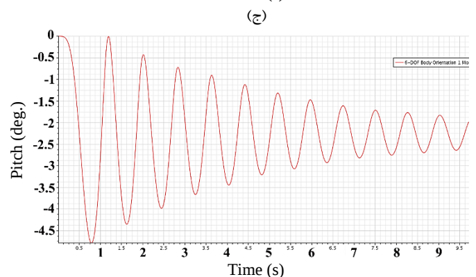
شکل ۱۸- نمودار حرکت پیچ شناور با پایدار ساز هیدروفویلی ساده در سه نسبت عرض و طول کورد مختلف؛
