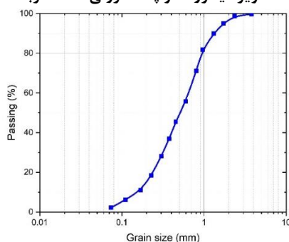
شکل ۲. منحنی توزیع اندازه ذرات ماسه کربناته کیش
