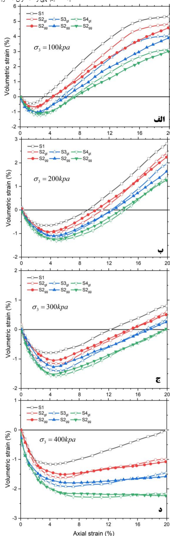
شکل ۶. منحنی‌های کرنش حجمی - کرنش محوری در تنش‌های همه‌جانبه مختلف
