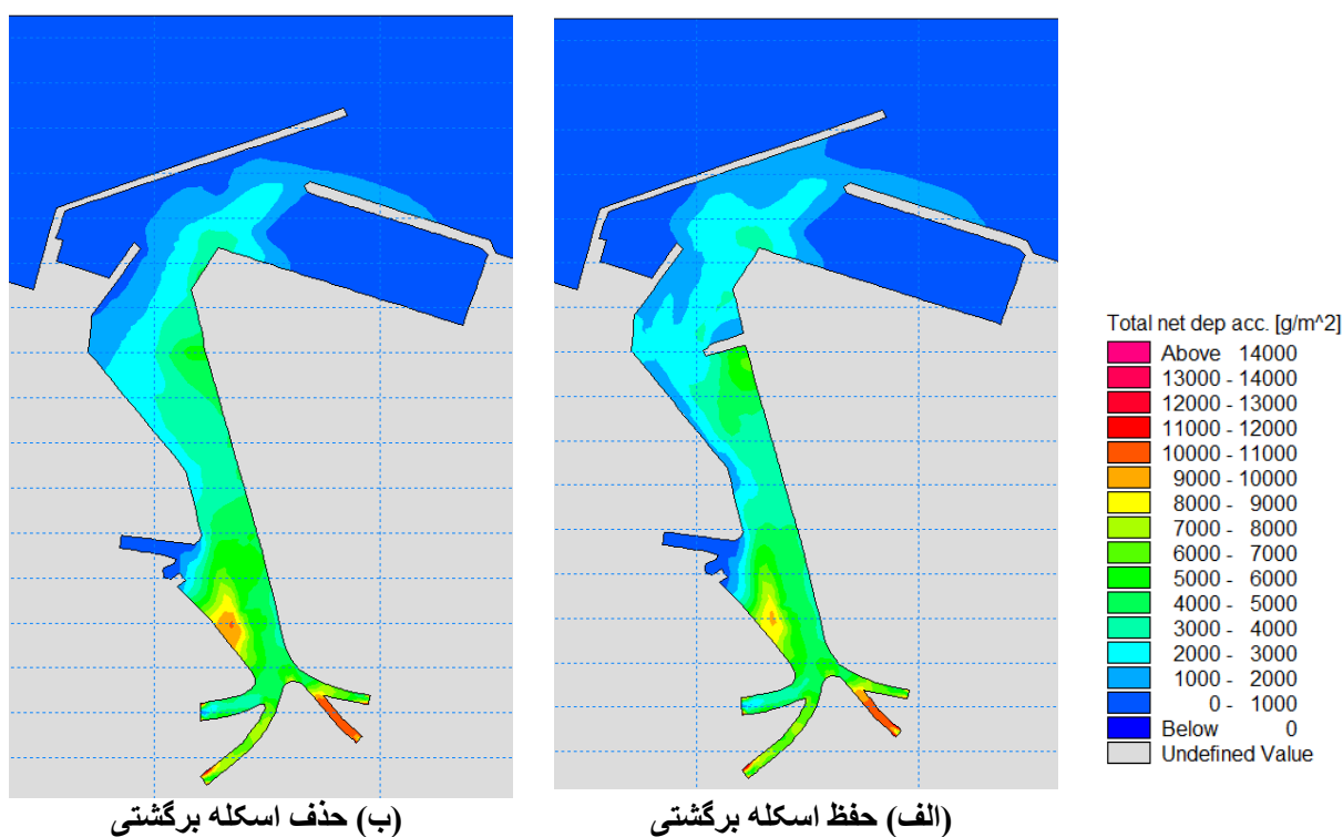
شکل ۱۴- الگوی نشست رسوبات در محدوده بندر در طول سیلاب متوسط
