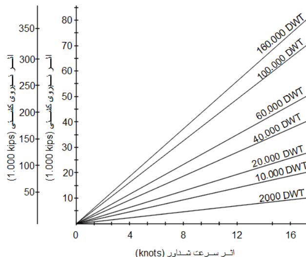
شکل ۲: اثر نیروی ناشی از برخورد شناور متناسب با سرعت شناور [۱۲]
