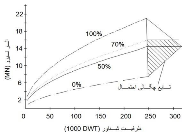
شکل ۴: توزیع احتمال نیروی ناشی از برخورد شناور [۱۲]
