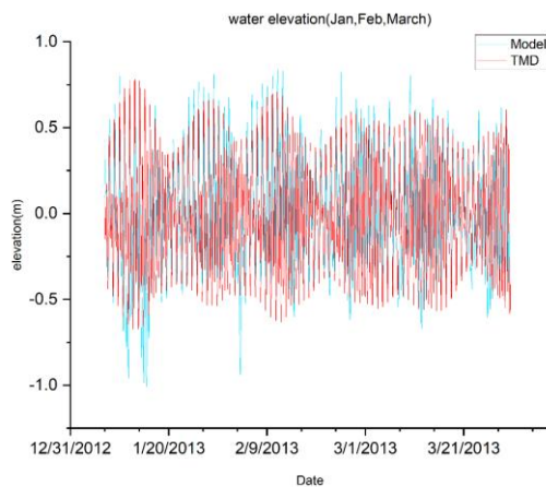
شکل ۵- مقایسه نتایج حاصل از مدل ROMS با داده‌های TMD در خلیج فارس در نزدیک ایستگاه فرزاد در شرط مرزی Chapman_implicit
