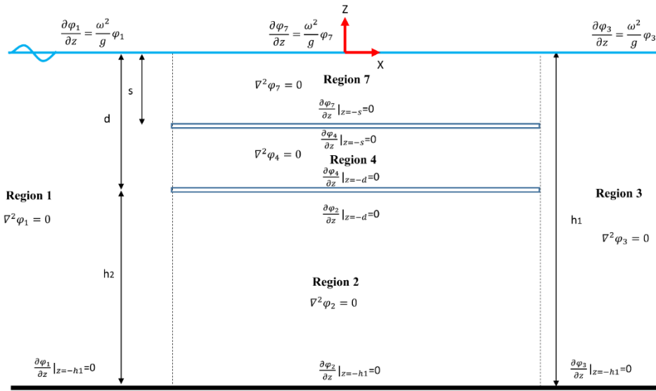
شکل ۳. شرط مرزی افقی مقطع A-A سکوی نیمه مغروق اصلاح شده با ورق میراگر دابل
