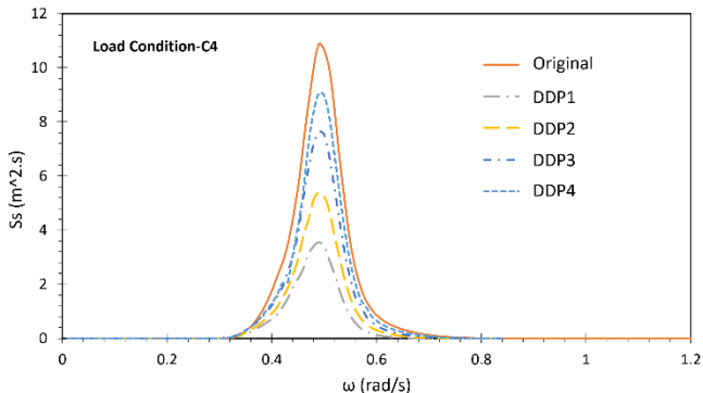
شکل ۲۳. پاسخ سکو اصلاح شده با شرایط موج C4
