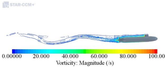
شکل ۸- ورتیسسته اطراف شناور
