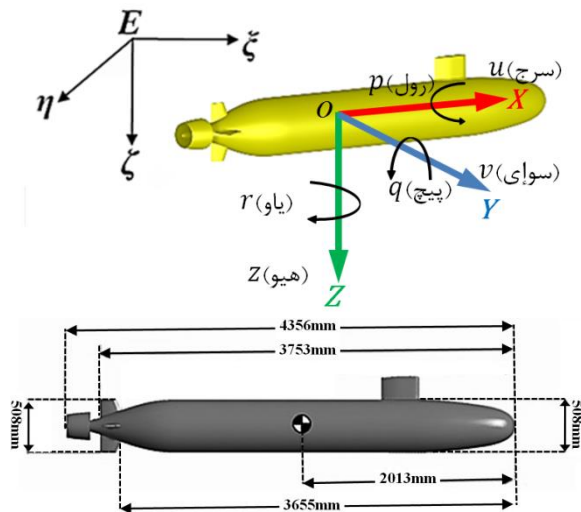
شکل ۱- ابعاد و هندسه سابوف، سیستم های مختصات بدنه و اینرسیایی، جهت و پارامترهای معادلات ۶ درجه آزادی
