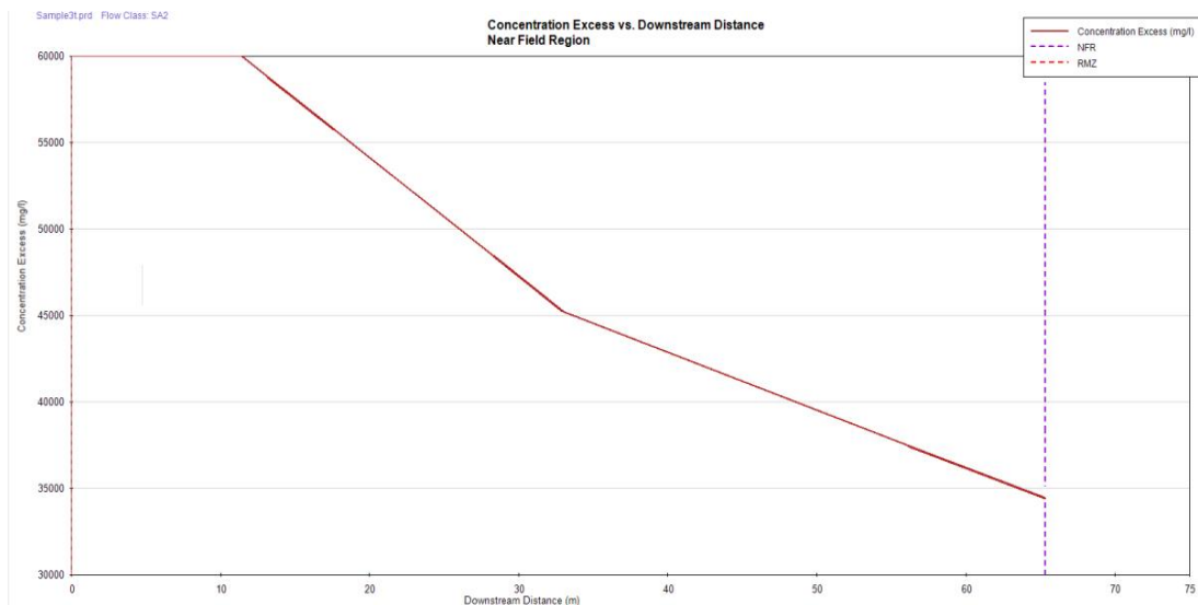
شکل ۱۰- غلظت در محدوده اختلاط میدان نزدیک برای دبی ۳ مترمکعب بر ثانیه با سرعت جریان حداکثر ۰/۰۵۷ متر بر ثانیه بعد از ۲ ساعت پس از اسلک
