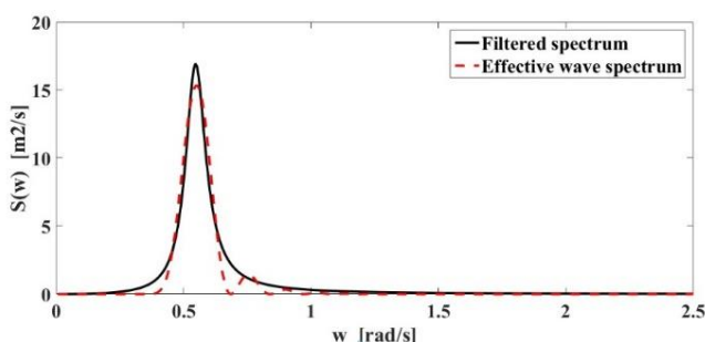
شکل ۴: طیف موج مؤثر و طیف موج فیلتر شده در حالت ارتفاع موج برابر با ۱۰/۴۳ متر و دوره تناوب پیک ۹/۹۹ ثانیه
