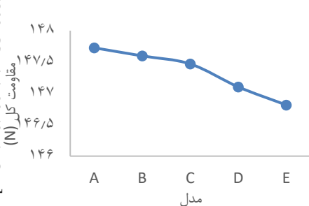
شکل ۱۶- نمودار مقاومت کل در عدد فرود ۰/۳۰
