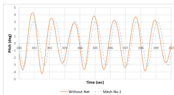
شکل ۱۳- مقایسه سری زمانی پیچ شناور مابین حالت ۳ و حالت ۶ مطابق با جدول ۵
