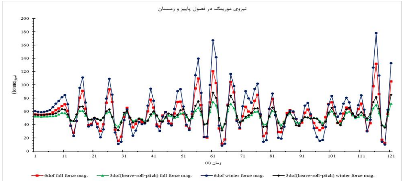
شکل ۱۳ - تاریخچه زمانی نیروهای مورینگ در دو حالت مدل سه درجه آزادی (هيو، رول و پیچ) و مدل شش درجه آزادی در فصل های پاییز و زمستان
