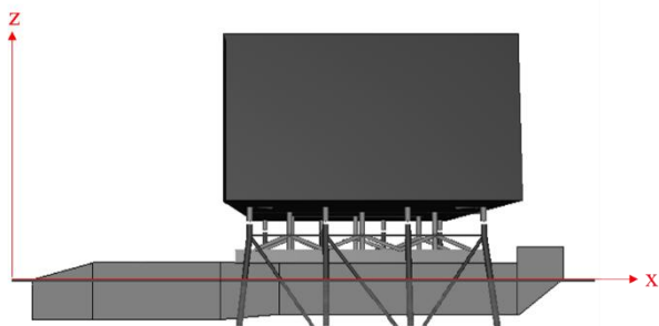
شکل ۲ - مدل شناور-سازه پشتیبیان-عرشه
