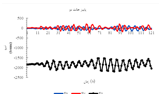
شکل ۹ - تاریخچه زمانی نیروهای وارده به المان میتینگ در فصل پاییز
