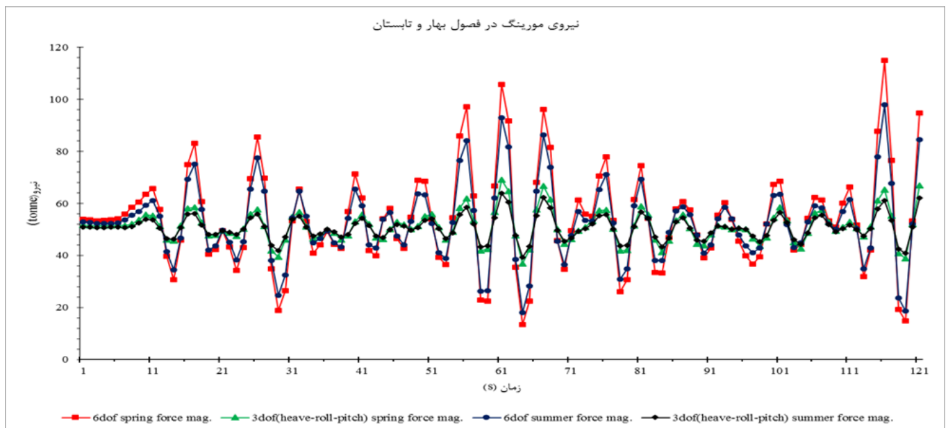
شکل ۱۲- تاریخیچه زمانی نیروهای مورینگ در دو حالت مدل سه درجه آزادی (هیو، رول و پیچ) و مدل شش درجه آزادی در فصل های پاییز و زمستان
