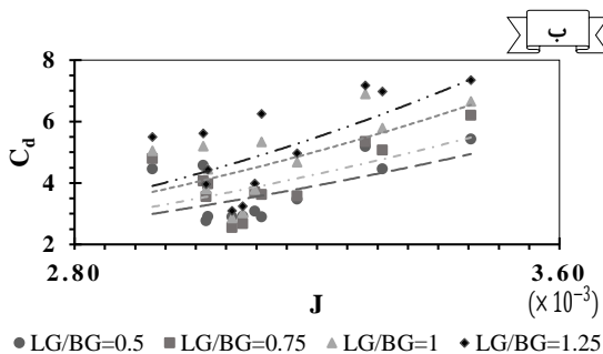
شکل ۹- الف: مستطیلی، ب: مثلثی) روند تغییرات ضریب پسا با شاخص صلبیت
