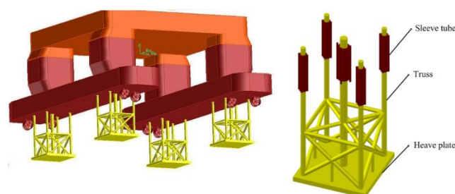
شکل ۳- ورق هیو در یک سکوی نیمه شناور [۸]
