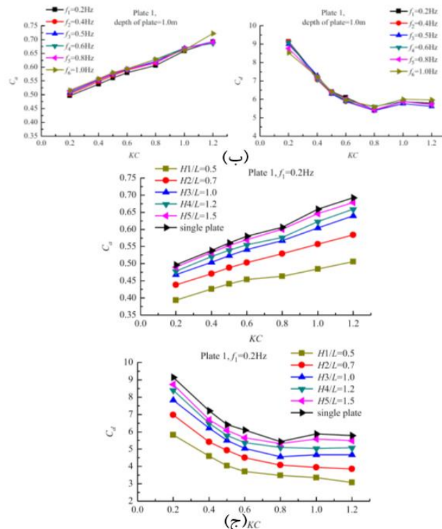
شکل ۱۵- (الف) نمای تجهیزات مورد استفاده (ب) تاثیر فرکانس (ج) تاثیر فاصله بین ورق‌ها روی ضرایب هیدرودینامیک [۴۹]
