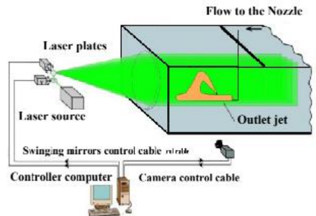
شکل ۱- نمای کلی از سامانه اسکن لیزری سه بعدی جهت آشکارسازی جریانات آغشته به فلورسنت [۲۰]
