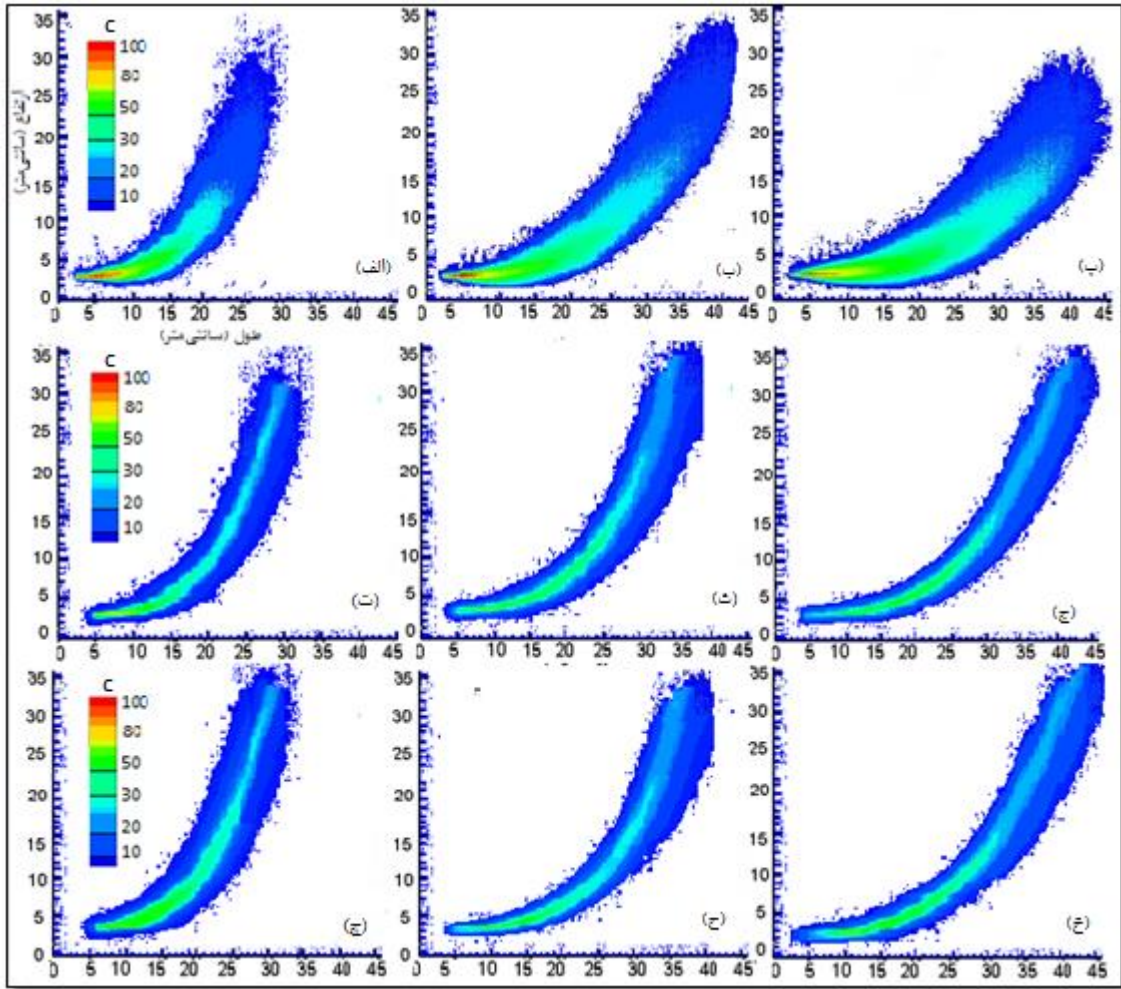
شکل ۴- مسیر حرکت جت، در مدل آزمایشگاهی (الف): Fr=10 ، (ب): Fr=15 و (پ): Fr=20 و در مدل آشفتگی k- \epsilon (ت): Fr=10 ، (ث): Fr=15 ، (ج): Fr=20 و در مدل آشفتگی RNG (چ): Fr=10 ، (ح): Fr=15 ، (خ): Fr=20
