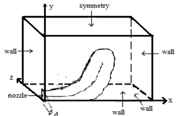
شکل ۲- نمای شماتیک از مسیر حرکت جت
