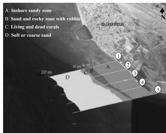
شکل ۲- محل ترانسکت‌های عمودی و عوارض بستر دریا [۶]
