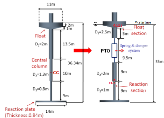
شکل ۱- سیستم مبدهل جاذب نقطه ای مبدهل انرژی امواج دریا (مدل لی و همکاران [۲۰])، سمت چپ: سیستم متشکل از یک جسم، راست: سیستم متشکل از دو جسم
