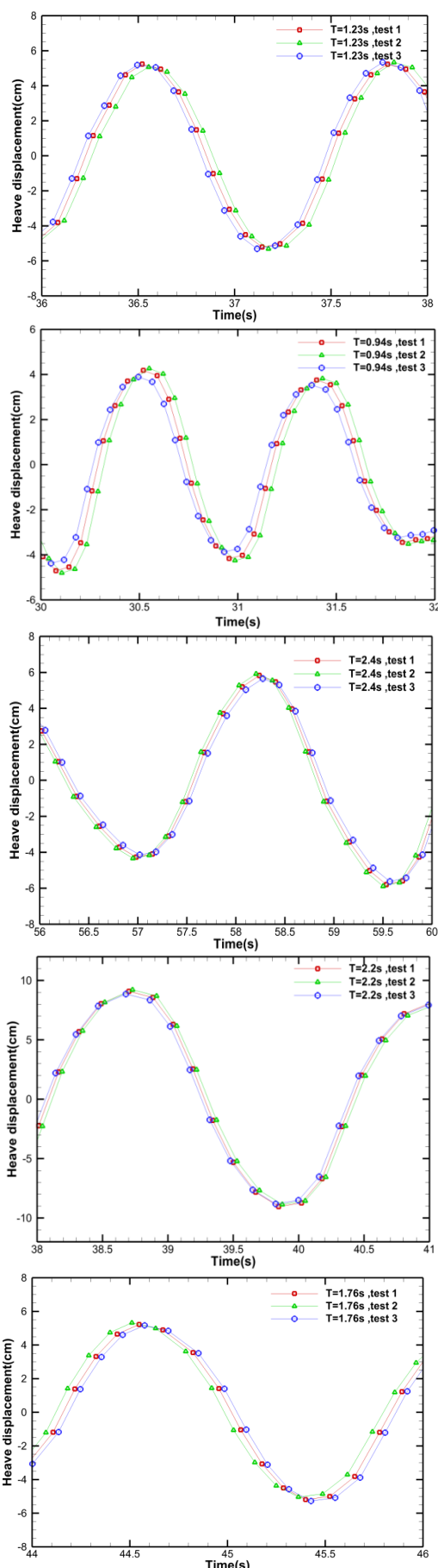
شکل ۱۱- مقایسه نتایج حاصل از تکرار آزمایش مدل (Test 1,2,3) در دوره تناوب T=0/94,1/23,1/76,2/2,2/4s
