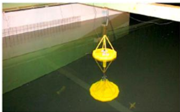
شکل ۴- تست مدل مبدل انرژی امواج دریا در آزمایشگاه برکلی (December 2010) [۱۳]
