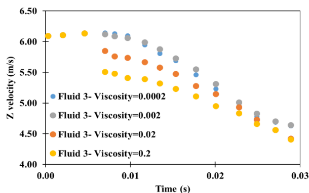
شکل ۴ - مقایسه تغییرات مقادیر سرعت حرکت گوه در سیال با توجه به تغییرات ثابت ویسکوزیته ( \text{pa.s}^N )
