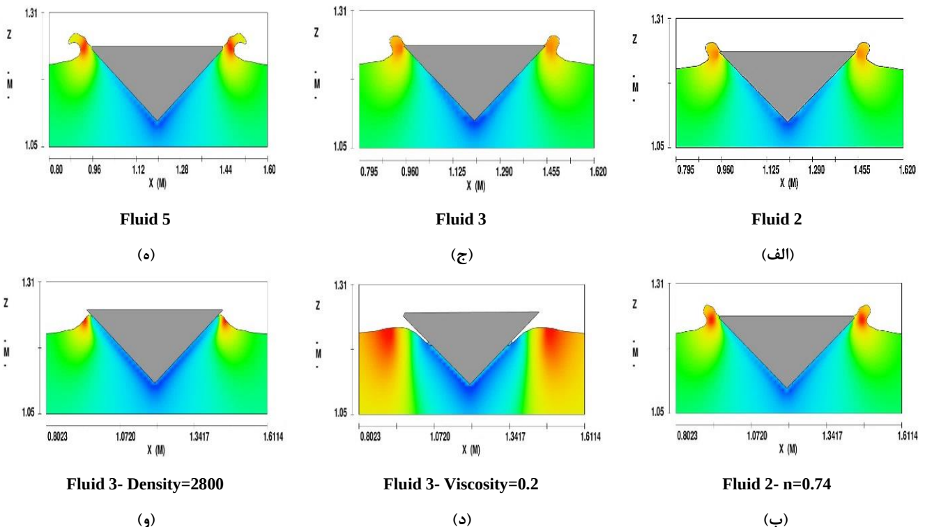
شکل ۶- مقایسه تغییرات سطح آزاد سیال در زمان t=0.024 ثانیه برای سیال‌های منتخب
