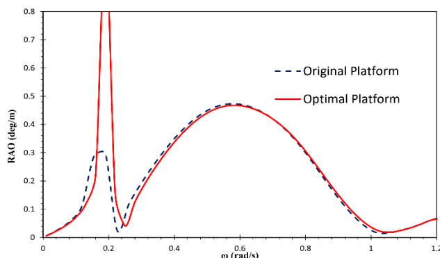
شکل ۱۱- مقایسه منحنی عملگر دامنه پاسخ حرکت پیچ سکوی نیمه مغروق امیر کبیر اجرا شده با نتایج حاصل از الگوریتم جستجوی شبکه‌ای
