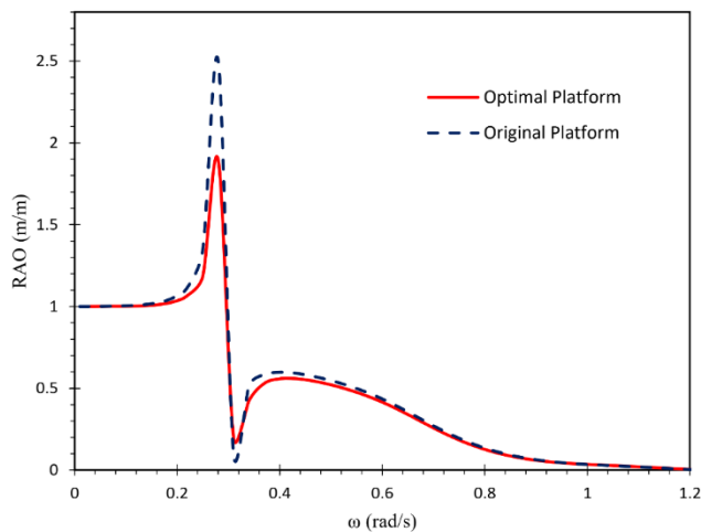
شکل ۱۰- مقایسه منحنی عملگر دامنه پاسخ حرکت هیو سکوی نیمه مغروق امیر کبیر اجرا شده با نتایج حاصل الگوریتم جستجوی شبکه‌ای
