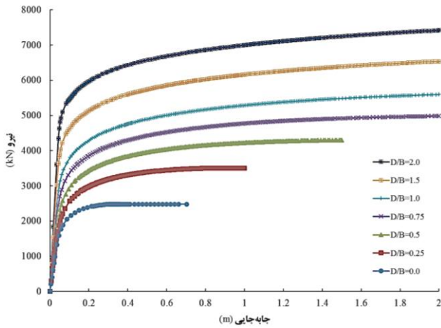
شکل ۵- نمونه‌ای از منحنی‌های پاسخ نیرو- جابه‌جایی پی لبه‌دار به‌ازای نسبت‌های مختلف عمق لبه (B=10 m, kB/sum=0, α=1)
