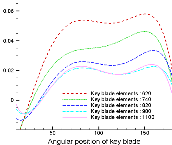
شکل ۱۱- تغییرات ضریب تراست پره اصلی در یک دور چرخش (از ورود به آب تا خروج) بر حسب ضریب پیشروی در J=0.5 تعداد مختلف المان‌ها در J=0.5
