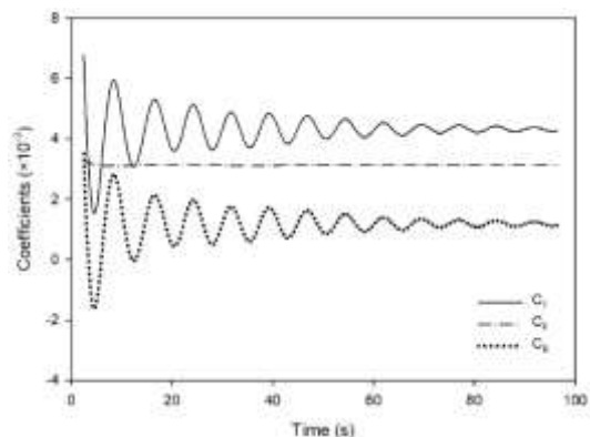
شکل ۱۶- ضرایب مقاومت کشتی ایران بوشهر
