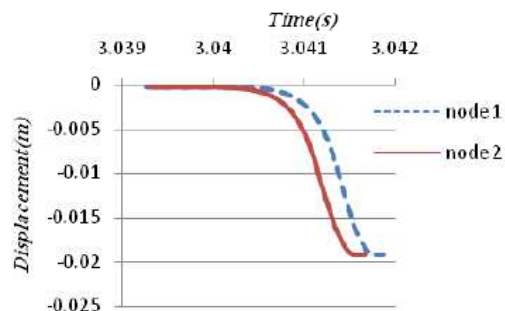
شکل ۷- نمودار تاریخچه زمانی جابجایی برای دو گره انتخابی روی مدل
