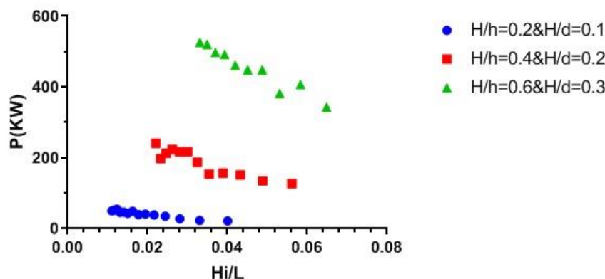
شکل ۱۶- تغییرات توان موج برخوردی به سازه با تیزی موج
