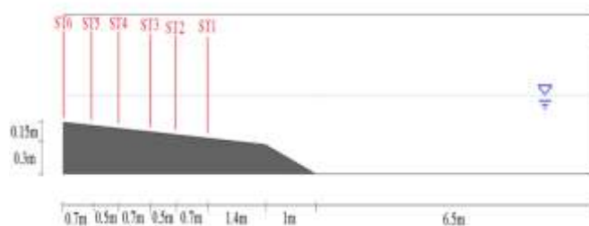
شکل ۱: موقعیت قرارگیری حسگرهای موج بر روی بستر شیب‌دار در کانال موج دو بعدی
