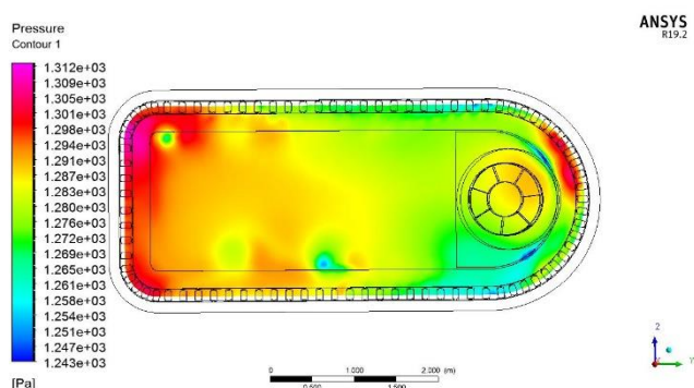
شکل ۳۱- کانتور توزیع فشار برای کانال ۴۵ درجه
