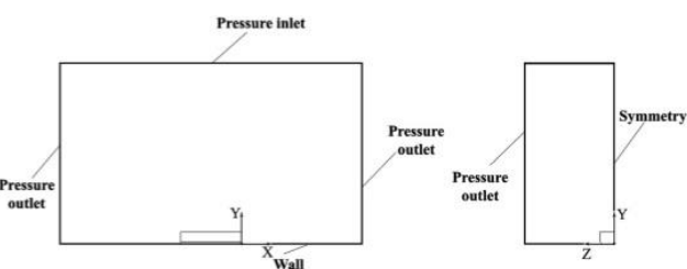
شکل ۲- دامنه حل و شرایط مرزی مسئله
