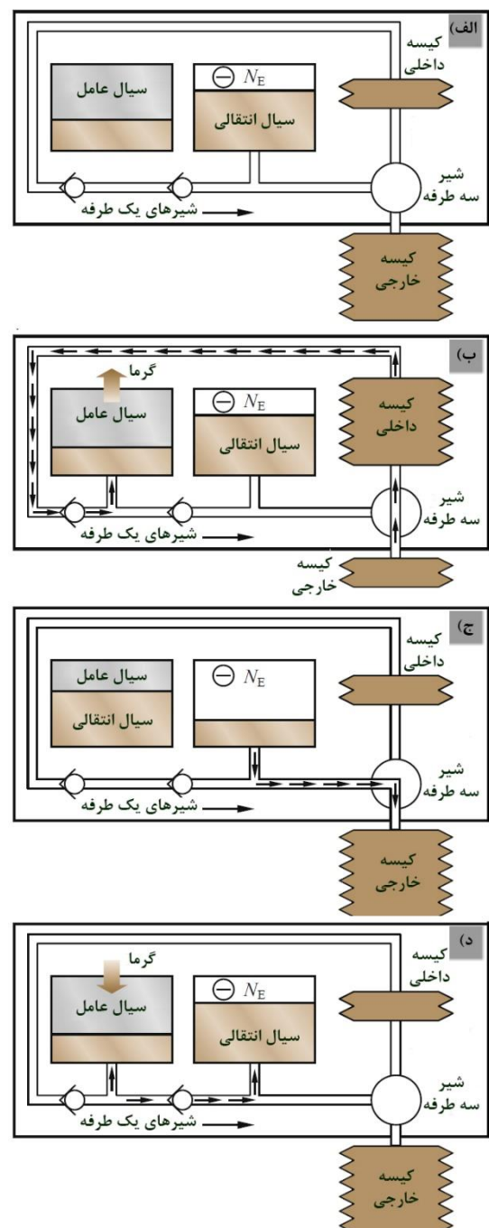
شکل ۳- حجم کنترلی ثابت و متغییر شناور
