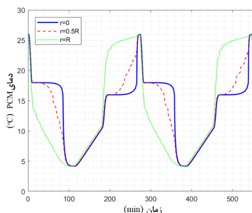
شکل ۱۲- تغییرات دمای هگزادکان با زمان در سه شعاع مختلف از محفظه حین فرآیند غوص و صعود
