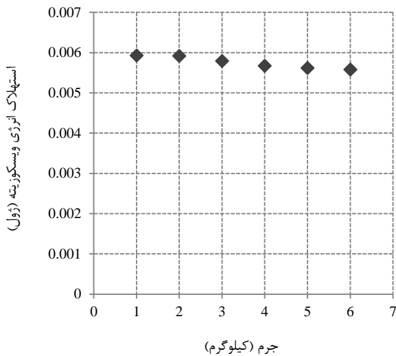
شکل ۱۵- تغییرات استهلاک انرژی و اسکوزیتنه بر حسب جرم پرتابه
