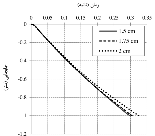
شکل ۳- مقایسه تاثیر اندازه مش‌بندی اوپلرین بر نمودار جابجایی - زمان پرتابه
