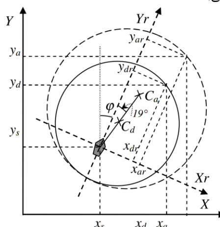
شکل ۷- دامنه و پهنه ایمن Davis
