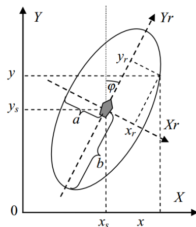
شکل ۹- دامنه ایمن بیضی شکل Fujii
