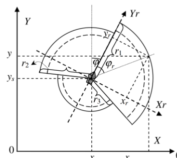
شکل ۶- دامنه ایمن دایره‌ای Goodwin
