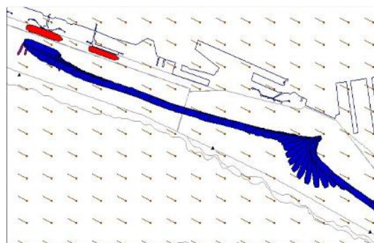
شکل ۴- مطالعه انجام شده توسط نرم‌افزار SHIPMA در آرژانتین [۱۹]
