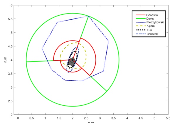
شکل ۱۴- مقایسه میان مدل‌های دایره ایمن (مایل دریایی)
