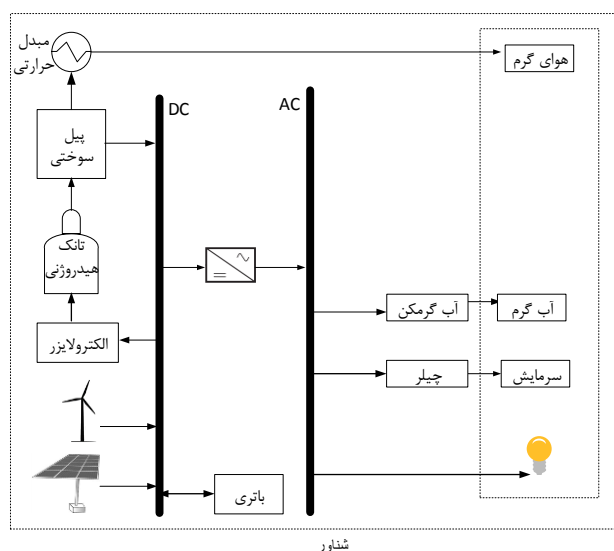
شکل ۱. ریزشکه پیشنهادی
