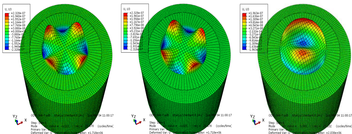
شکل ۱۶- اشکال مودی ورق دایره‌ای با ضخامت ۰/۱ متر در تماس با سیال آب
