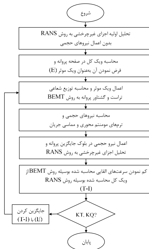
شکل ۵ - الگوریتم حل ترکیبی RANS/BEMT
