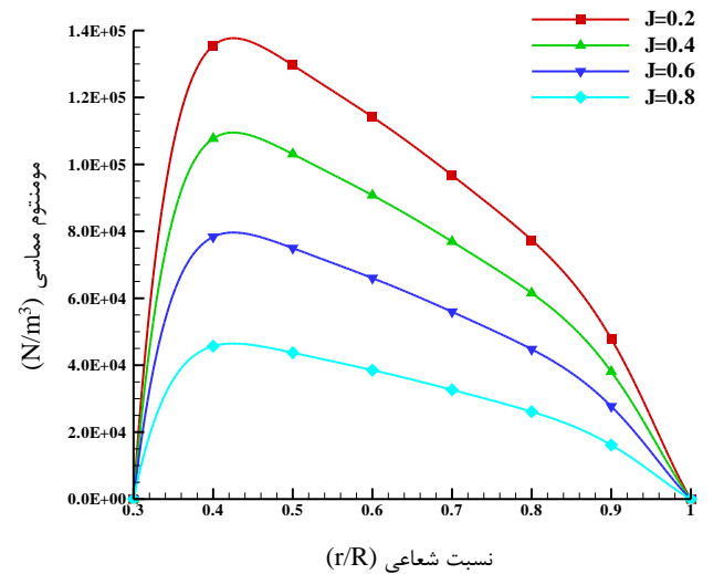
شکل ۱۳- مقادیر ترم‌های مومنتوم مماسی به روش BEMT
