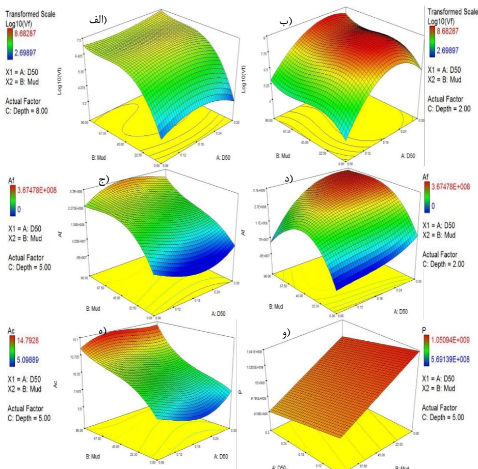
شکل ۵- مدل‌سازی آماری پاسخ‌های حوضچه به تغییرات پارامترهای مورفولوژیک رسوبات چسبنده و d_{50} (الف) V_f در عمق حداکثر ۸ متر ب) V_f در عمق حداقل ۲ متر ج) A_f در عمق حداکثر ۵ متر د) A_f در عمق حداقل ۲ متر ه) سطح مقطع عرضی کانال Ac و حجم منشور جزر و مدی P
