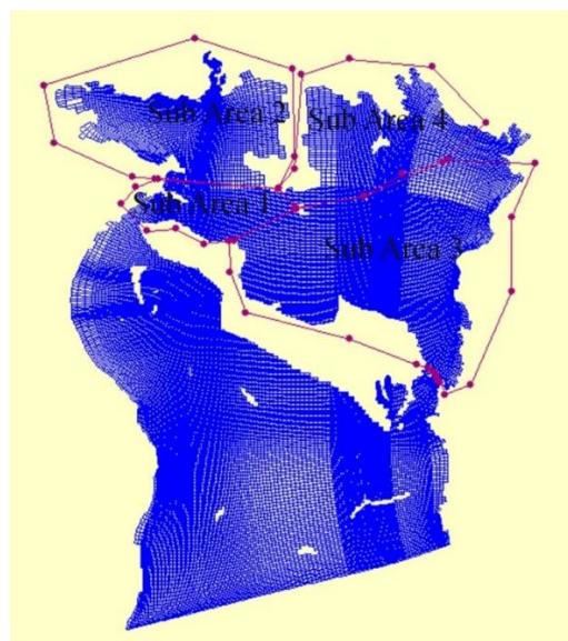
شکل ۲- شبکه بندی مستطیلی خور موسی که در محیط Delft3D تهیه شده است. تعداد بهینه سلول ها تعادل بین هزینه محاسباتی و دقت مدلسازی بلند مدت پدیده های مهم را برقرار می نماید.
