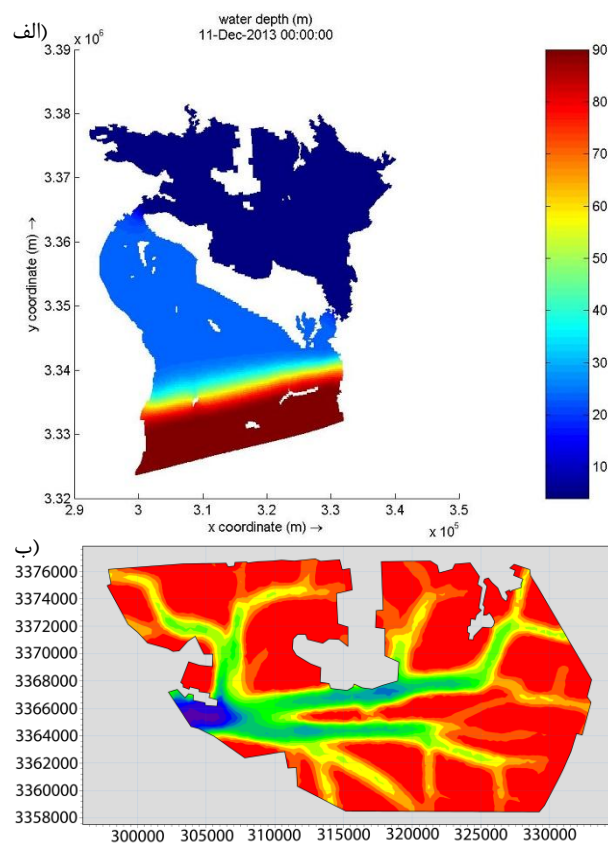
شکل ۴-الف) هیدروگرافی شماتیک اولیه برای مدل‌سازی درون حوضچه از یک بتیمتری مسطح با عمق ۴ m استفاده شده است که توسط یک بتیمتری با شیب ملایم به خلیج فارس متصل شده است. ب) بتیمتری اندازه‌گیری شده در سال ۱۳۸۳ درون حوضچه خور موسی.
