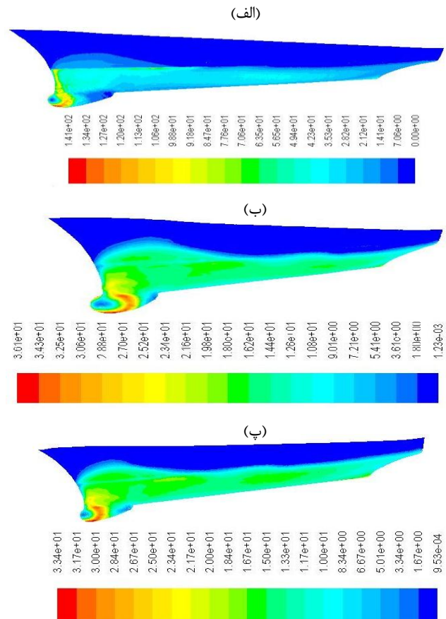
شکل ۱۵ - مقایسه تنش برشی وارد بر بدنه شناور با سرعت جریان آزاد ۳/۰۷۱ m/s در فرود ۰/۴۱، (الف): شناور در حالت خزه گرفتگی آهکی شدید، (ب): شناور با پوشش سیلیکونی، (پ): شناور با پوشش کوپلیمر مسی
