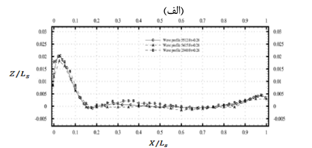
شکل ۷- معتبر سازی پروفایل موج روی سطح بدنه شناور در فرود ۰/۲۸، (الف): موج تجربی، (ب): موج عددی
