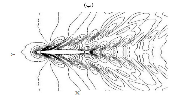
شکل ۵- مقایسه انتشار موج مدل سازی شده در سطح آزاد شناور ۵۴۱۵ با مقادیر تجربی فرود ۰/۲۸، (الف): موج تجربی، (ب): موج عددی
