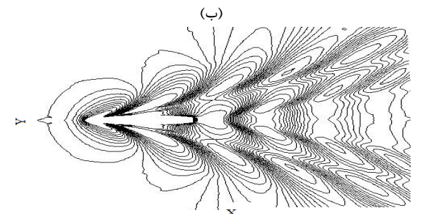
شکل ۷- معتبر سازی پروفایل موج روی سطح بدنه شناور در فرود ۰/۲۸، (الف): موج تجربی، (ب): موج عددی
