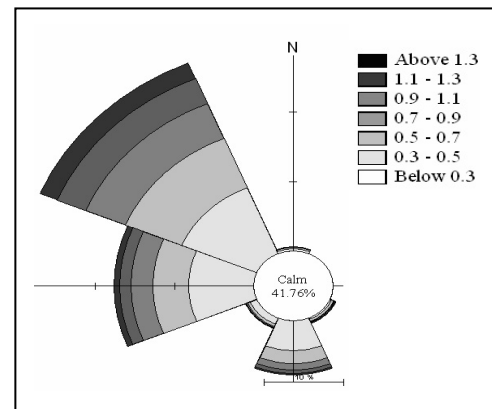
شکل ۱۴- گلموج دو ساله حاصل از مدلسازی عددی (بندر بوشهر)
