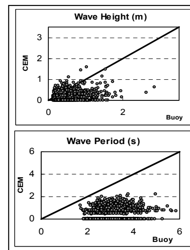
شکل ۵ - مقایسه مقادیر اندازه‌گیری شده و پیش‌بینی شده ارتفاع و دوره تناوب موج توسط روش CEM (منطقه امیرآباد)
