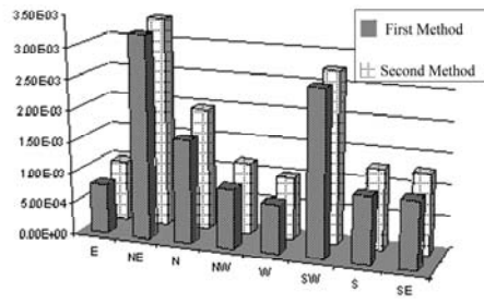
شکل ۱۴- مقایسه احتمال خرابی محاسبه شده با روش اول و دوم و ضریب تغییرات بارگذاری برابر ۵ درصد (سکوی P.2)
