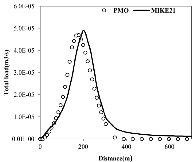
شکل ۱۱- مقایسه بار کل رسوب شبیه سازی شده در PMO و MIKE21 در ساحل شرقی (چپ) و غربی (راست) موج ۱/۵ متر
