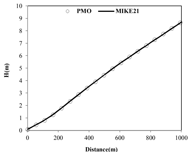
شکل ۹- مقایسه سرعت جریان و عمق آب شبیه سازی شده در PMO و MIKE21 در ساحل غربی موج ۱/۵ متر
