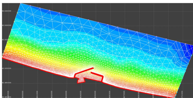
شکل ۳- شبکه بندی محدوده شبیه سازی شده
