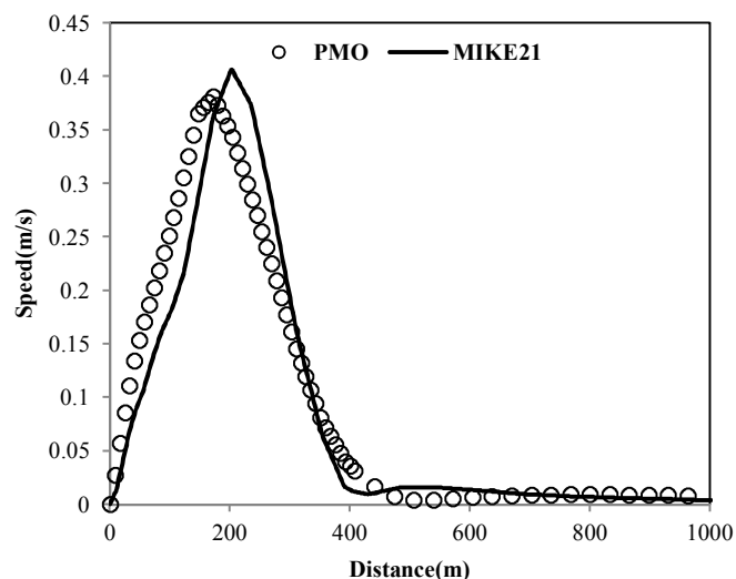
شکل ۹- مقایسه سرعت جریان و عمق آب شبیه سازی شده در PMO و MIKE21 در ساحل غربی موج ۱/۵ متر
