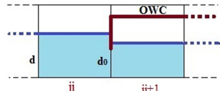
شکل ۲ - دو سلول مجاور ستون نوسان‌گر آب
