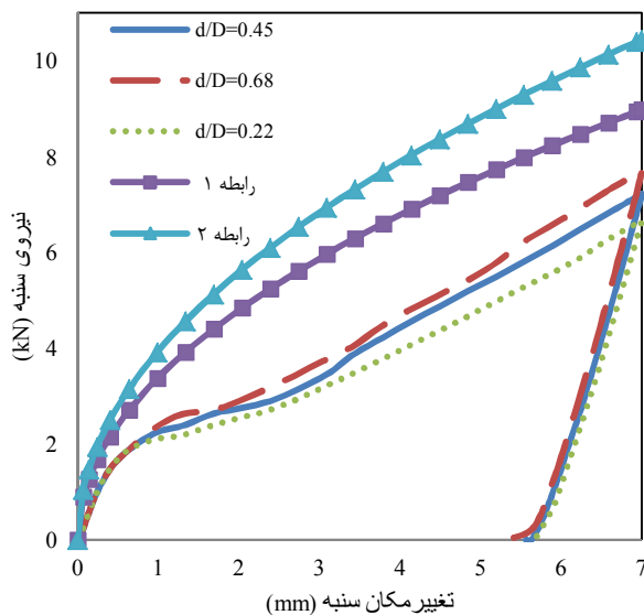
شکل ۱۶- تاثیر نسبت d/D بر مقاومت جانبی لوله‌ای
