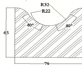
شکل ۲- مقطع هندسی بلوک بستر لوله (واحد mm). طول بلوک برابر با ۶۵ میلیمتر است.
