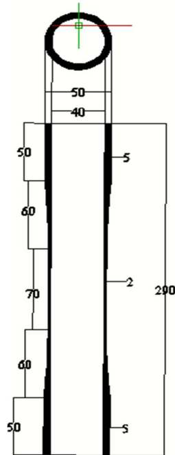
شکل ۱- مشخصات هندسی نمونه‌های آزمایشگاهی (واحد mm)
