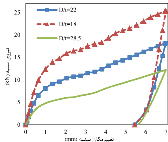
شکل ۱۴- تاثیر نسبت D/t بر مقاومت جانبی لوله
