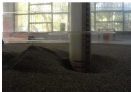
(ب): طوقه به فاصله ۵۰ سانتی‌متر
