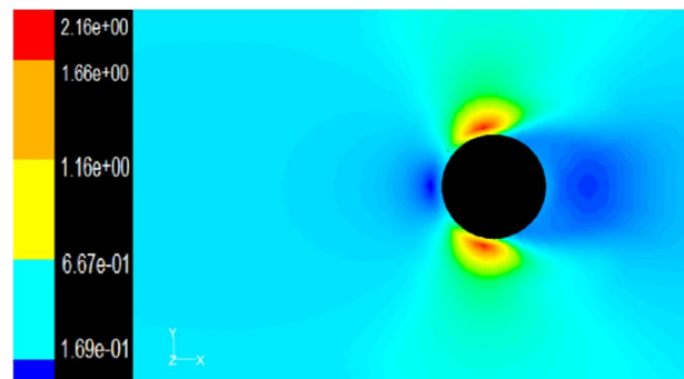
(الف): طوقه به فاصله ۷/۵ سانتی‌متر از بستر
