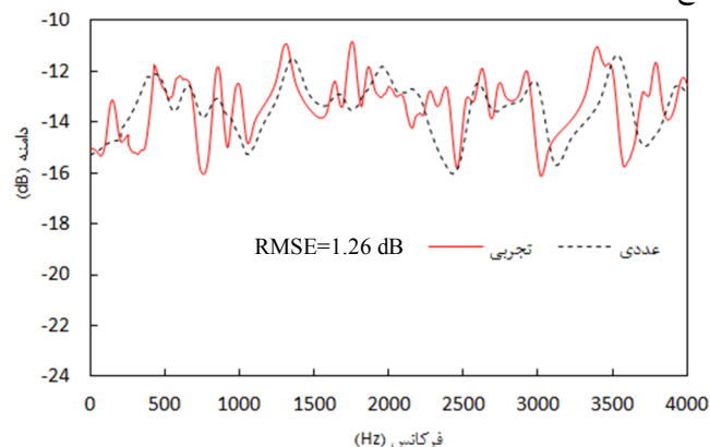
شکل ۳- مقایسه دامنه توابع پاسخ فرکانسی سیستم اولیه برای سه
