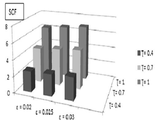
شکل ۲۴- تأثیر ناکاملی هندسی عضو مهاریهی روی SCF در Crown 180° ( \alpha = 12^\circ , \beta = 0.6 , \theta = 90^\circ , \gamma = 10 )
