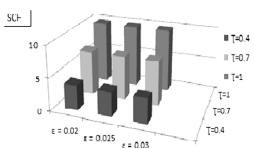
شکل ۱۰- تأثیر ناکاملی هندسی عضو مهارى روی SCF در ( \alpha = 12, \theta = 90^\circ, \beta = 0.3, \gamma = 10 ) Saddle
