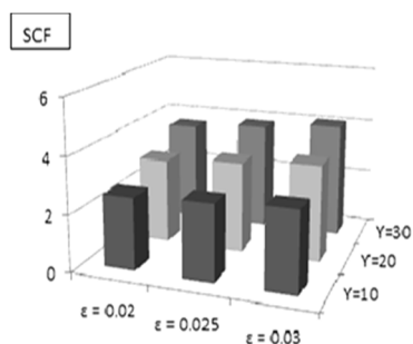
شکل ۲۰- تأثیر ناکاملی هندسی عضو مهاري روی SCF در ( \alpha = 12, \beta = 0.3, \theta = 90^\circ, \tau = 0.4 ) Crown 180°
