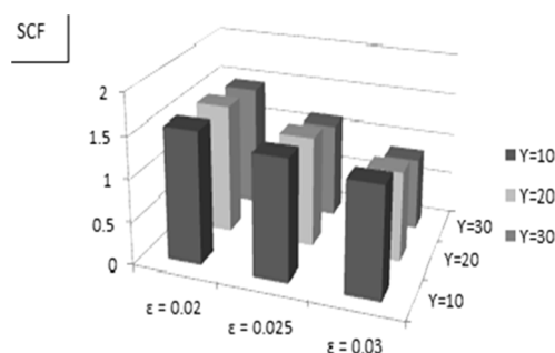
شکل ۱۳- تأثیر ناکاملی هندسی عضو مهارى روی SCF در ( \alpha = 12, \beta = 0.3, \theta = 90^\circ, \tau = 0.4 ) Crown 0^\circ
