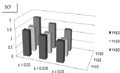
شکل ۱۴- تأثیر ناکاملی هندسی عضو مهارى روی SCF در ( \alpha = 12, \beta = 0.45, \theta = 90^\circ, \tau = 0.4 ) Crown 0^\circ
