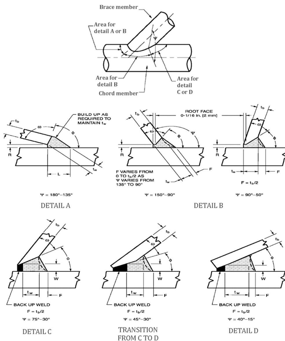
شکل ۳- جزئیات پروفیل جوش مطابق با ضوابط AWS D1.1 [۱۴]
