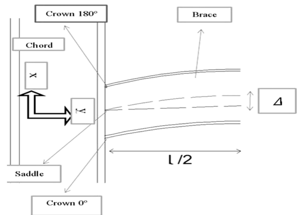
شکل ۱- نمونه‌ای از مدل با ناکاملی هندسی عضو مهار
