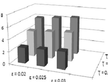
شکل ۲۳- تأثیر ناکاملی هندسی عضو مهاري روی SCF در ( \alpha = 12, \beta = 0.45, \theta = 90^\circ, \gamma = 10 ) Crown 180°
