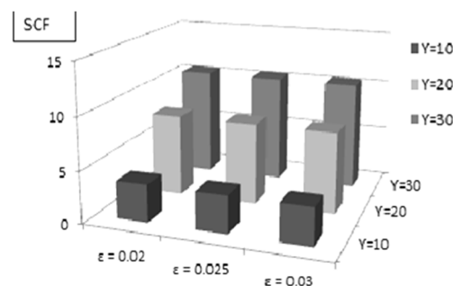
شکل ۹- تأثیر ناکاملی هندسی عضو مهارى روی SCF در ( \alpha = 12, \beta = 0.6, \theta = 90^\circ, \tau = 0.4 ) Saddle
