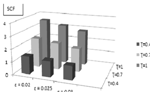
شکل ۱۸- تأثیر ناکاملی هندسی عضو مهاري روی SCF در ( \alpha = 12, \beta = 0.6, \theta = 90^\circ, \gamma = 10 ) Crown 0°
