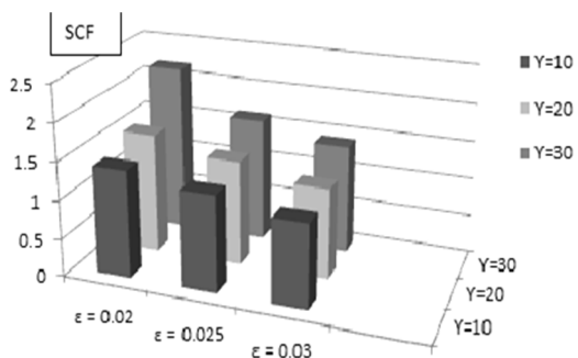
شکل ۱۵- تأثیر ناکاملی هندسی عضو مهارى روی SCF در ( \alpha = 12, \beta = 0.6, \theta = 90^\circ, \tau = 0.4 ) Crown 0^\circ
