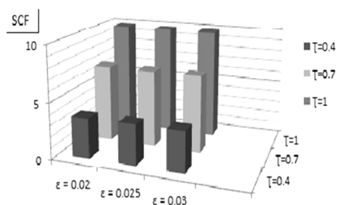
شکل ۱۲- تأثیر ناکاملی هندسی عضو مهارى روی SCF در ( \alpha = 12, \beta = 0.6, \theta = 90^\circ, \gamma = 10 ) Saddle
