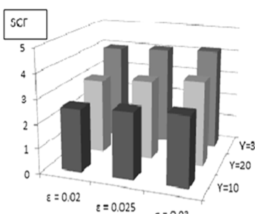
شکل ۲۱- تأثیر ناکاملی هندسی عضو مهاري روی SCF در Crown ( \alpha = 12, \beta = 0.3, \theta = 90^\circ, \tau = 0.4 ) 180°
