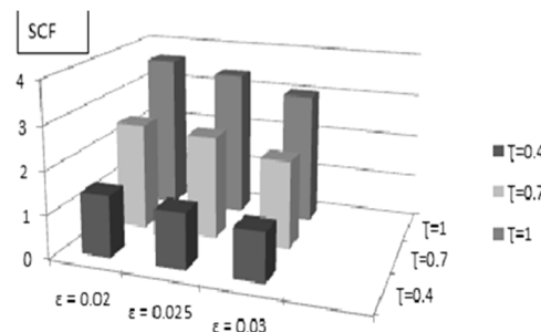
شکل ۱۷- تأثیر ناکاملی هندسی عضو مهاري روی SCF در ( \alpha = 12, \beta = 0.45, \theta = 90^\circ, \gamma = 10 ) Crown 0°
