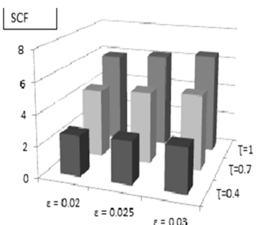
شکل ۲۲- تأثیر ناکاملی هندسی عضو مهاري روی SCF در ( \alpha = 12, \beta = 0.3, \theta = 90^\circ, \gamma = 10 ) Crown 180°
