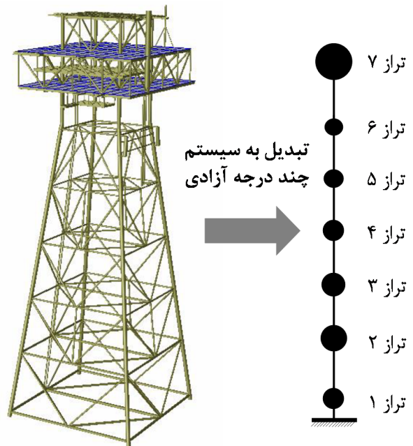
شکل ۵ - سکوی رسالت و مدل ساده شده چند درجه آزادی
