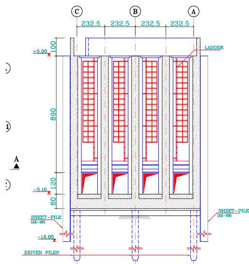
شکل ۲- دریچه های خروجی آب نیروگاه
