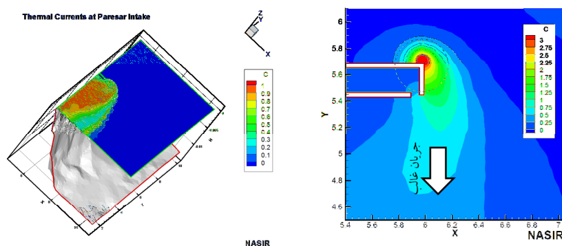
شکل ۱۲- دمای میانگین در اطراف خروجی نیروگاه پره سردر شرایط باد و بدون جریان غالب (واحدهای مختصات بر حسب کیلومتر می‌باشند)
