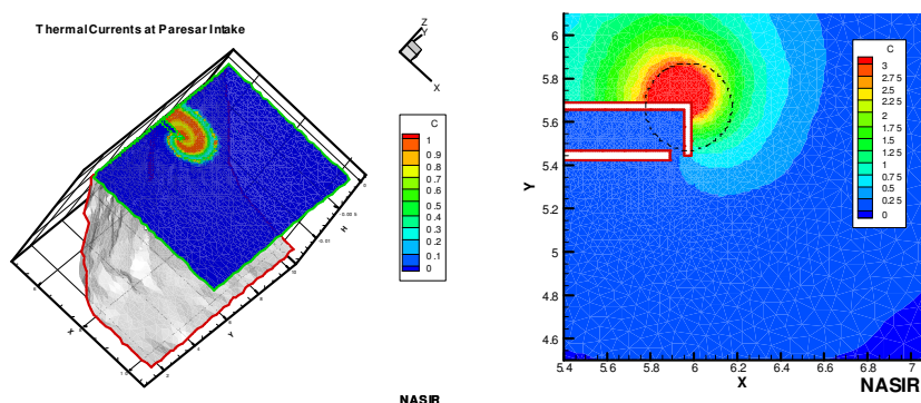
شکل ۱۳- دمای میانگین عمقی در اطراف خروجی نیروگاه پره سردر شرایط آرام (بدون باد و جریان) (واحدهای مختصات بر حسب کیلومتر می‌باشند)
