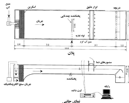
شکل ۵- هندسه و مشخصات کانال آزمایش [۲]
