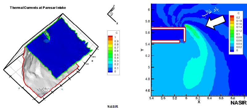
شکل ۱۱- دمای میانگین عمقی در اطراف خروجی نیروگاه پره سردر شرایط باد غالب و بدون جریان (واحدهای مختصات بر حسب کیلومتر می‌باشند)
