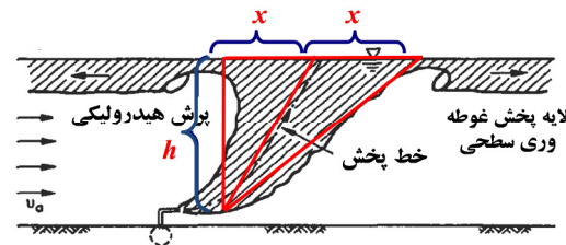
شکل ۳- محاسبه محدوده میدان نزدیک در اطراف خروجی نیروگاه پره سر با توجه به شکل پلوم
